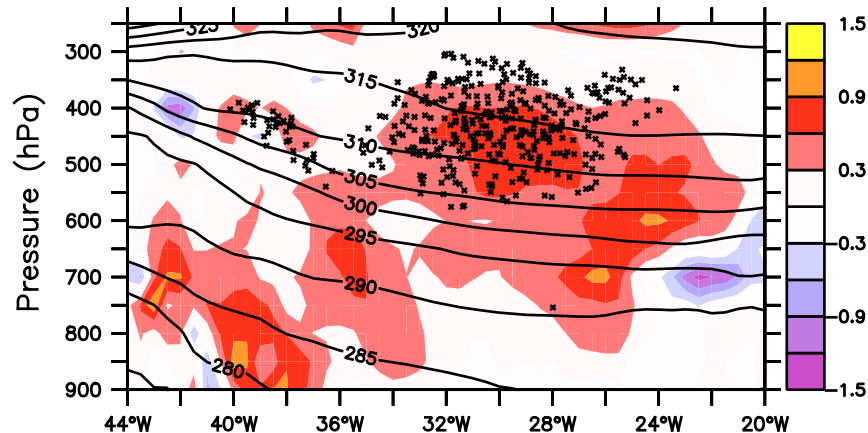
(d) PCMT, 63°N–65°N averaged heating (K/h)
