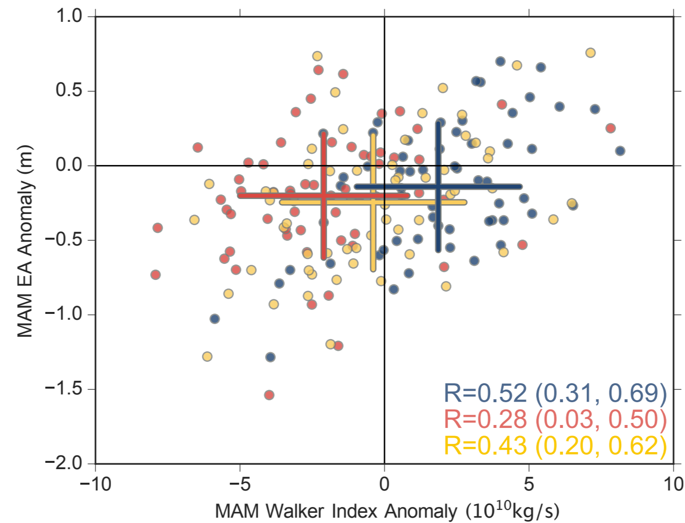
(b) MAM EA vs. MAM Walker
