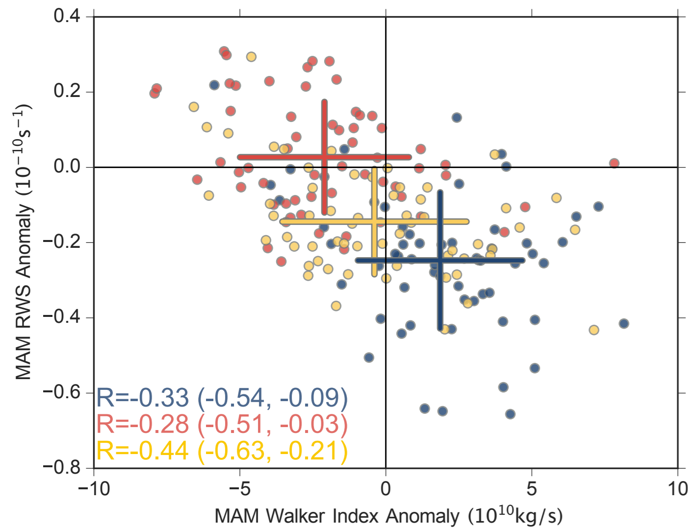
(a) MAM RWS vs. MAM Walker
