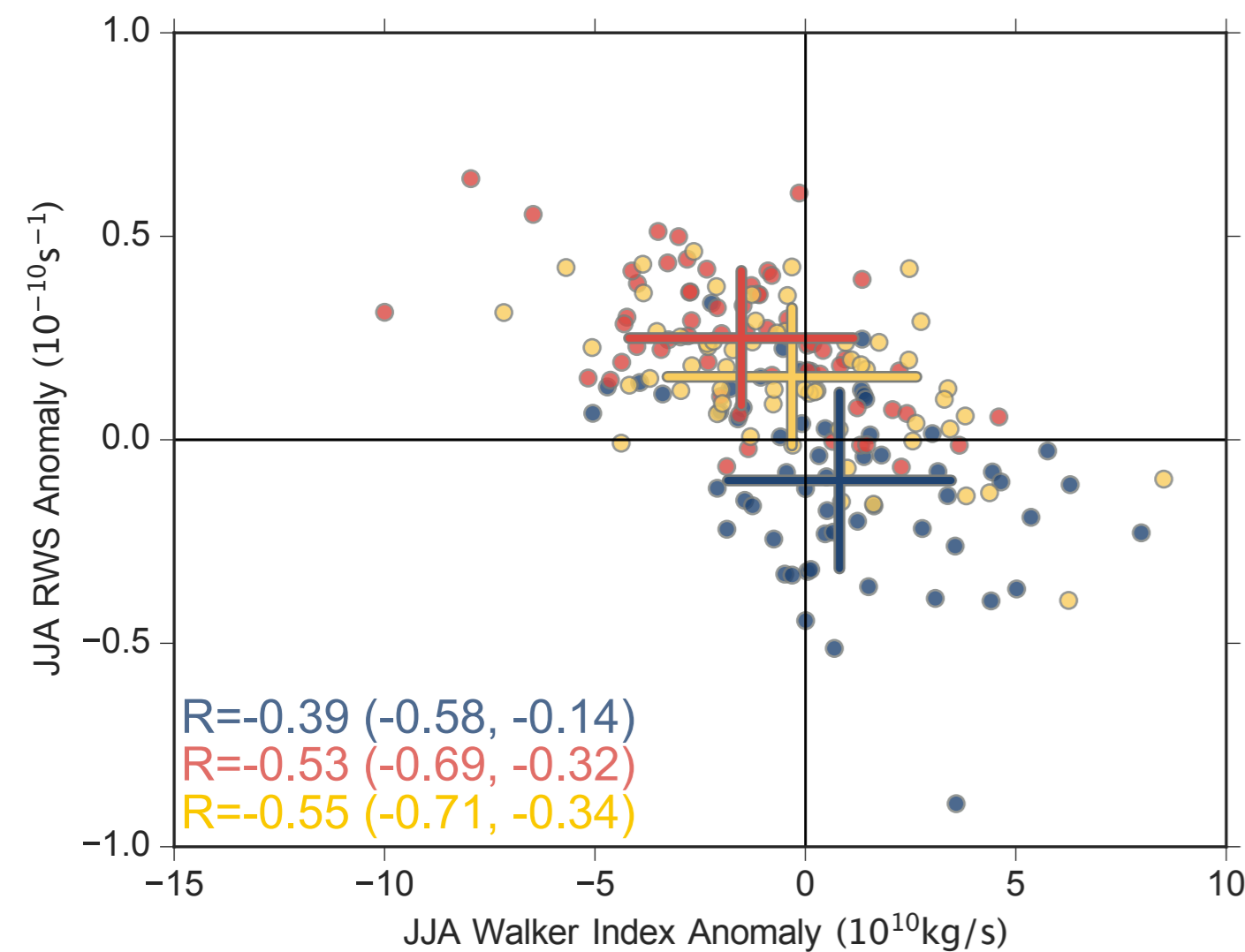
(d) JJA RWS vs. JJA Walker
