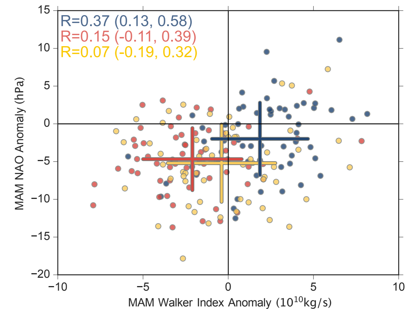
(c) MAM NAO vs. MAM Walker
