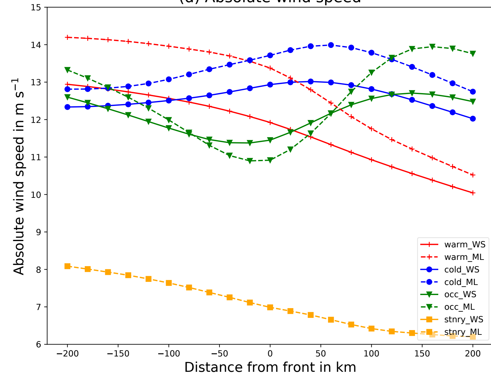
(d) Absolute wind speed
