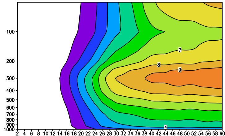
(d) Jan Spread U(m/s) (m=1–3) (60–90°N)
