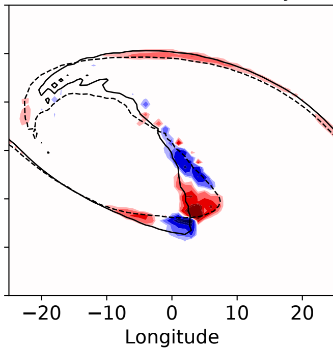
(d) Rotational wind tendency
