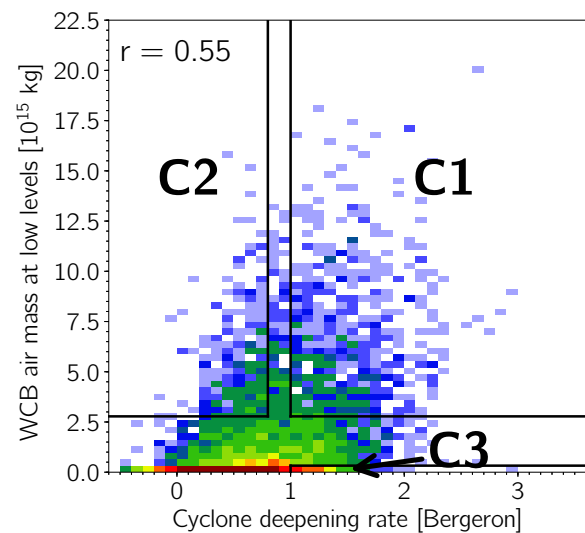
(f) CESM-RCP85, SH
