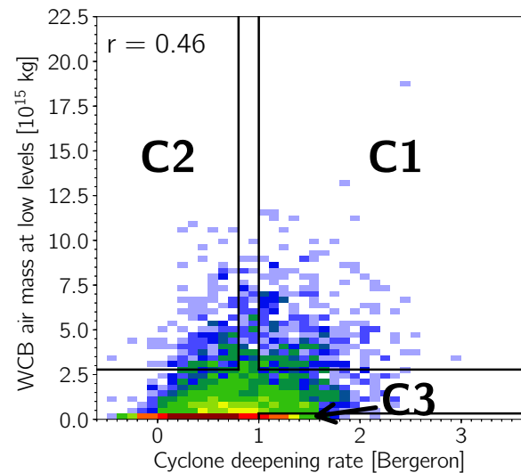
(d) CESM-HIST, SH
