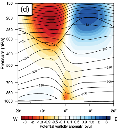
CESM-RCP85, SH
