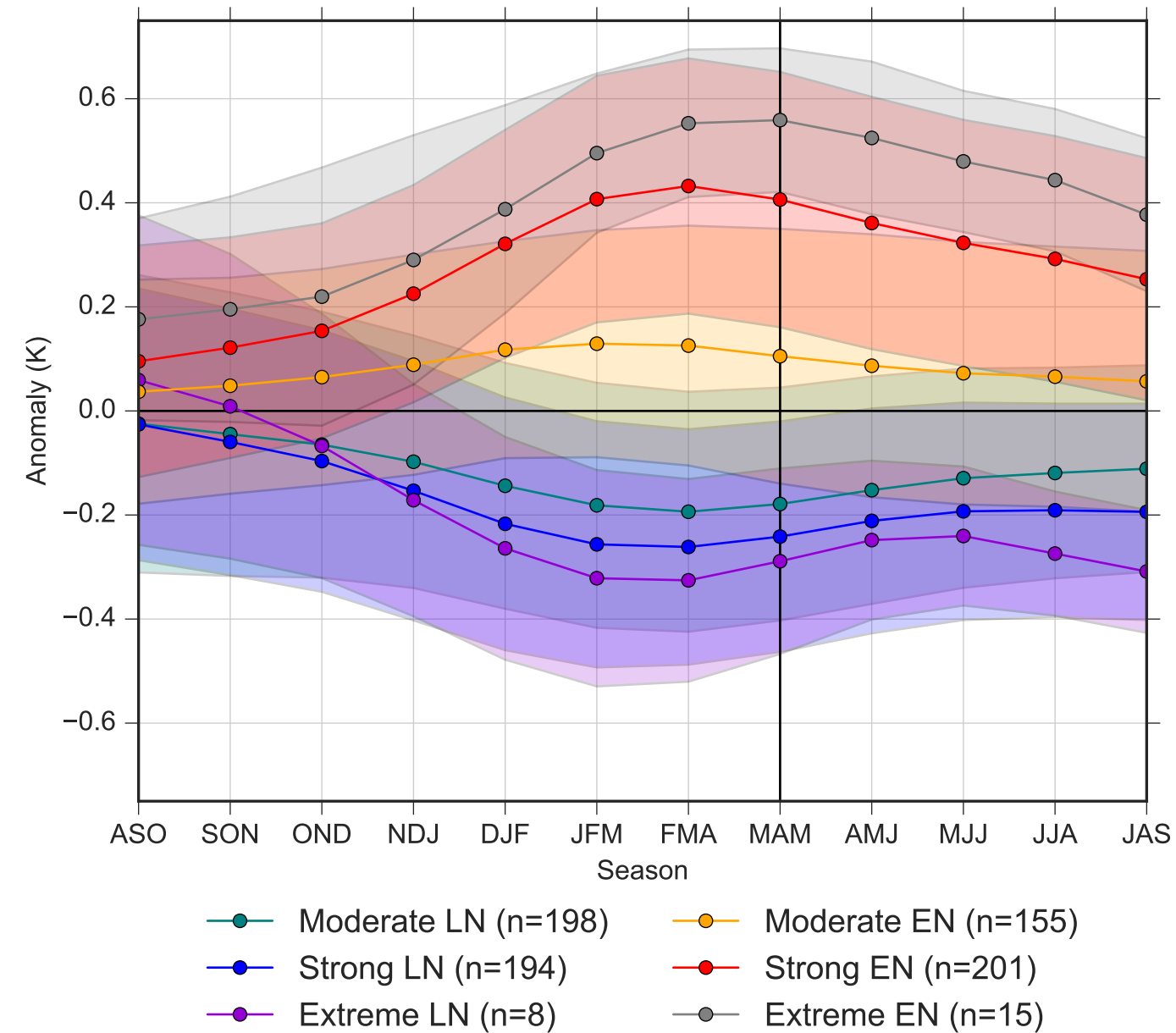
(a) TNA SSTA Evolution (CESM-WACCM)
