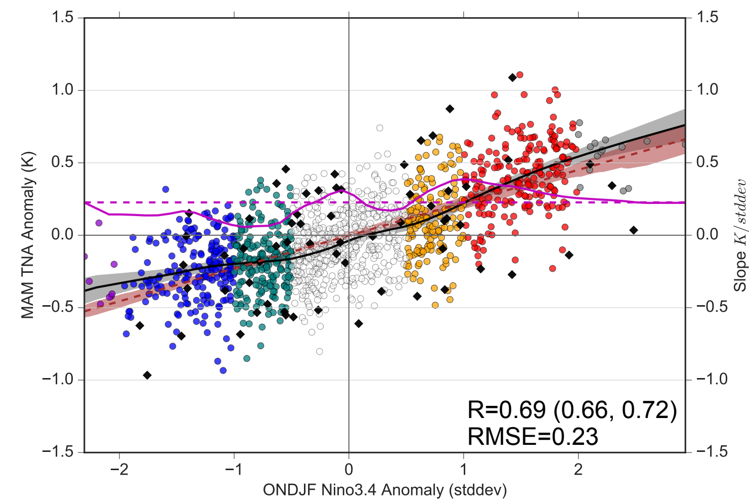
(c) MAM TNA SSTA (CESM-WACCM)
