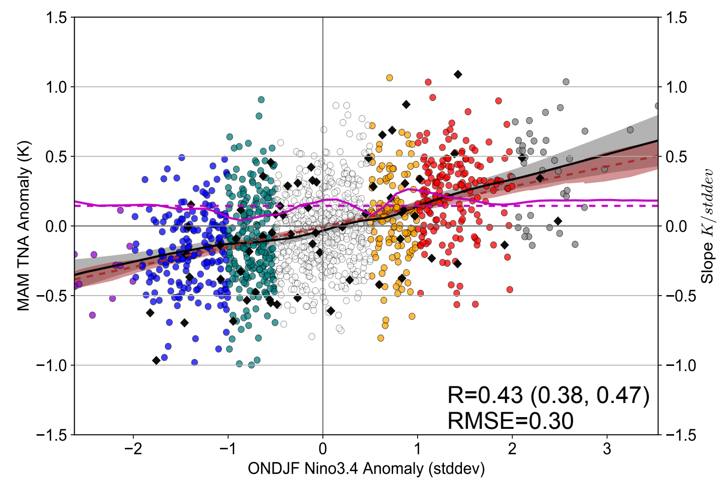
(d) MAM TNA SSTA (FOCI)
