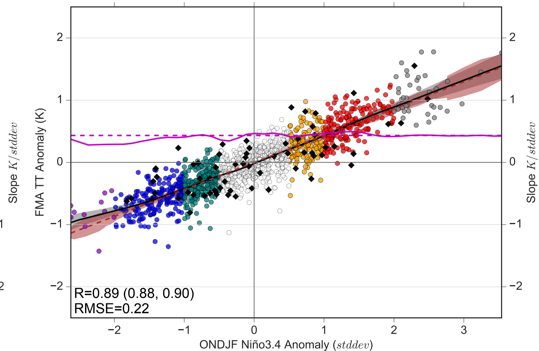
(d) Secondary Gill Response (FOCI)
