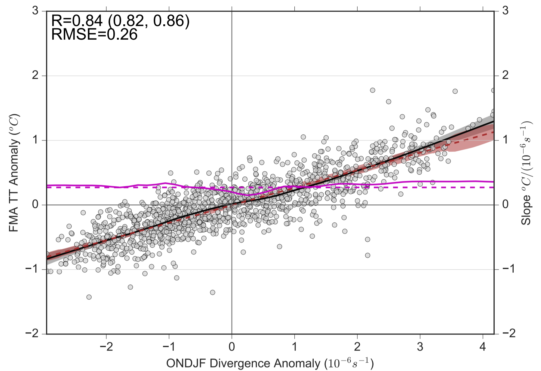
(d) FOCI 2Gill vs. 200 div. (159°E-160°W)
