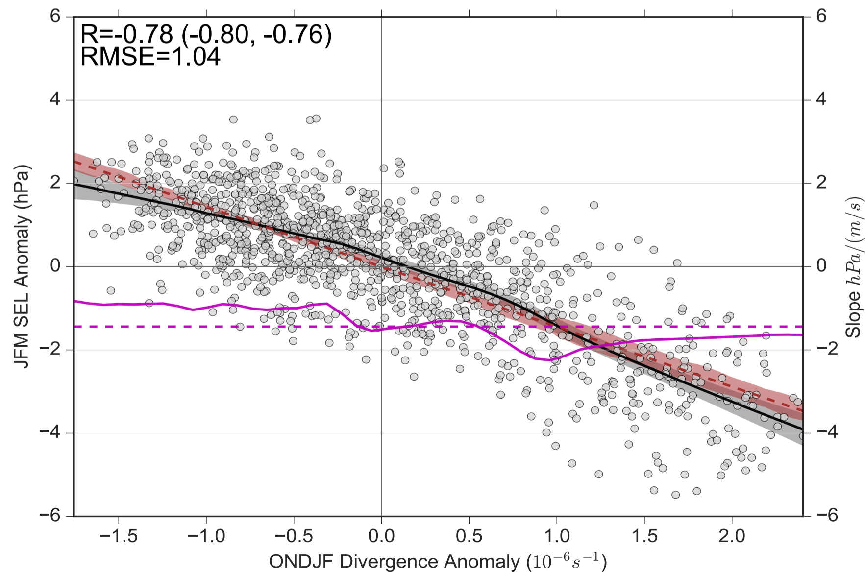
(e) CESM-WACCM SEL vs. 200 div. (137°E-115°W)
