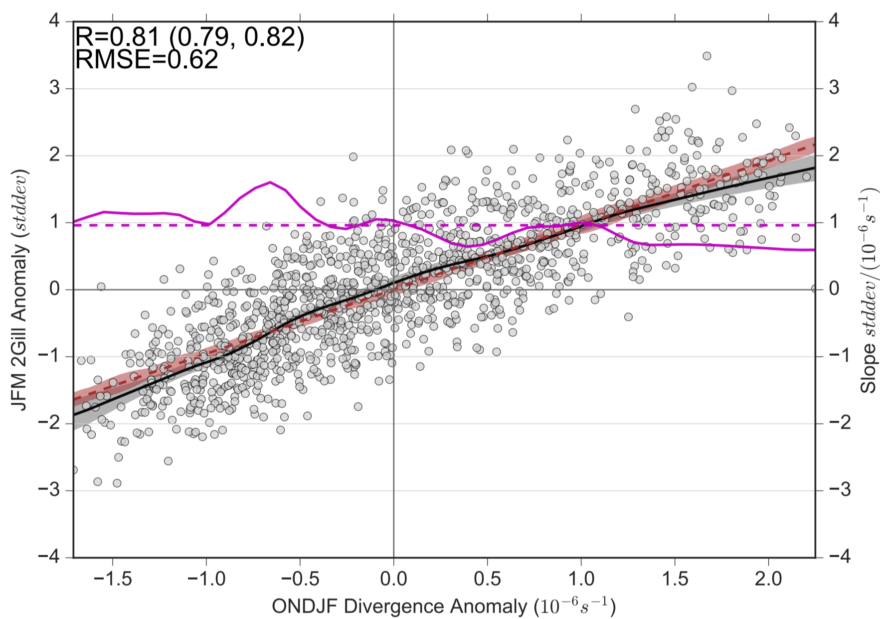
(e) CESM-WACCM SEL vs. 200 div. (137°E-115°W)
