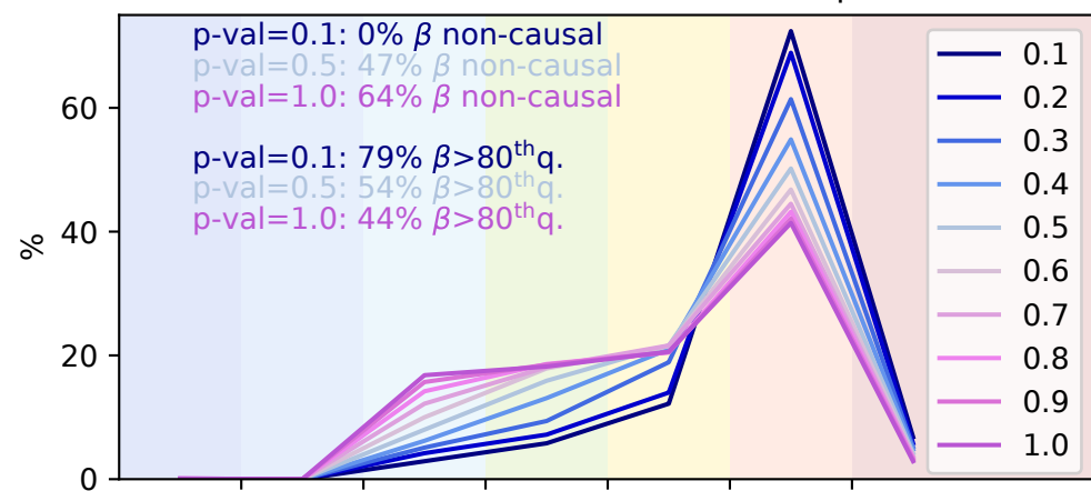
(b) All links, MCA1 SAM \Rightarrow Z200|CGT
