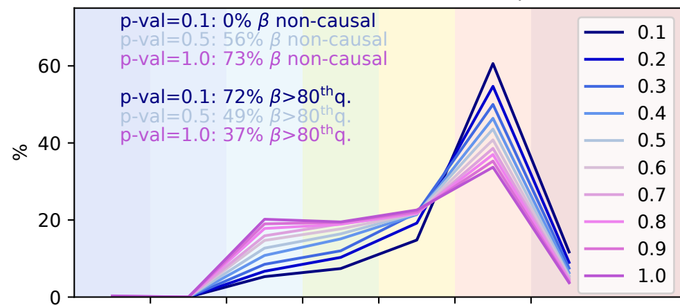
(d) All links, MCA1 SAM \Rightarrow OLR|CGT
