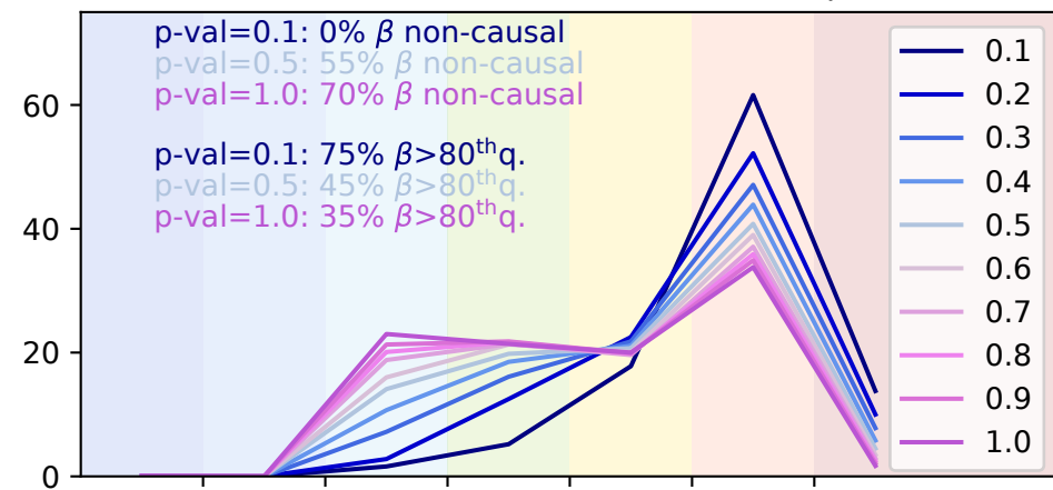
(g) All links, MCA2 NPH \Rightarrow OLR|WNPSM
