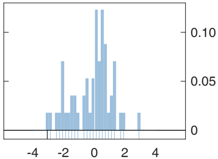
(b) 15 yr trends (ERA5)
