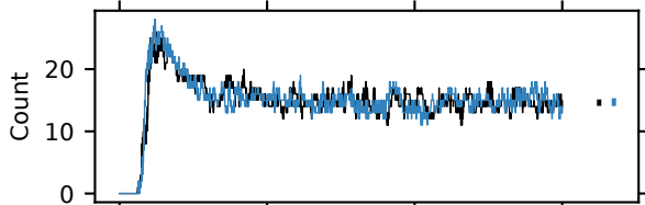
(d) Half-earth-radius TC world
