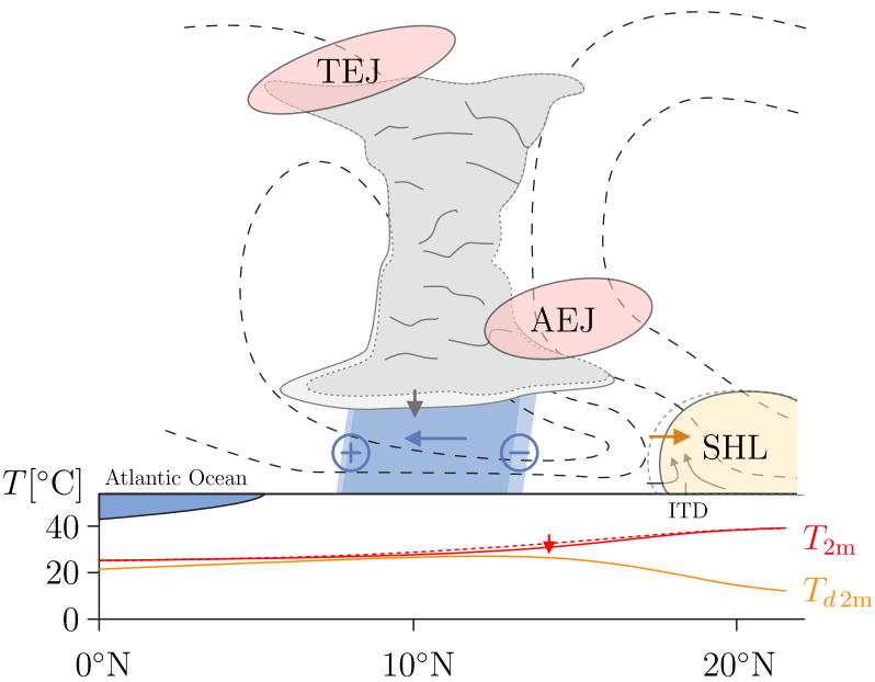
(b) rhebc_land_trop
