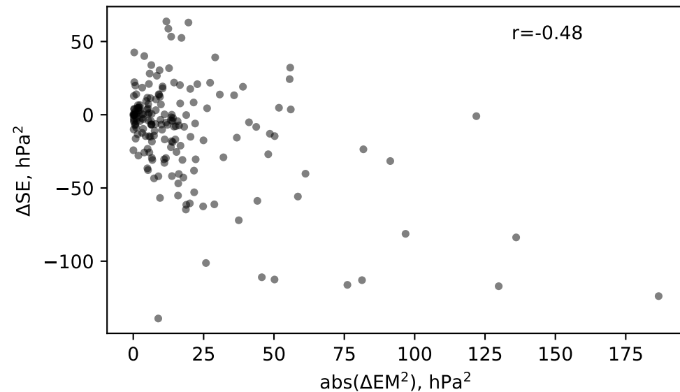
(d) Europe: \Delta SE vs \text{abs}(\Delta EM^2)
