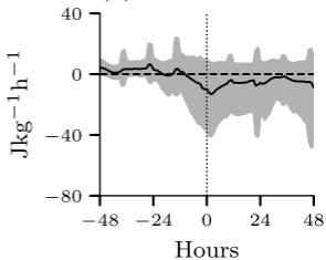
(d) Diabatic
