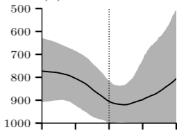
(d) Diabatic
