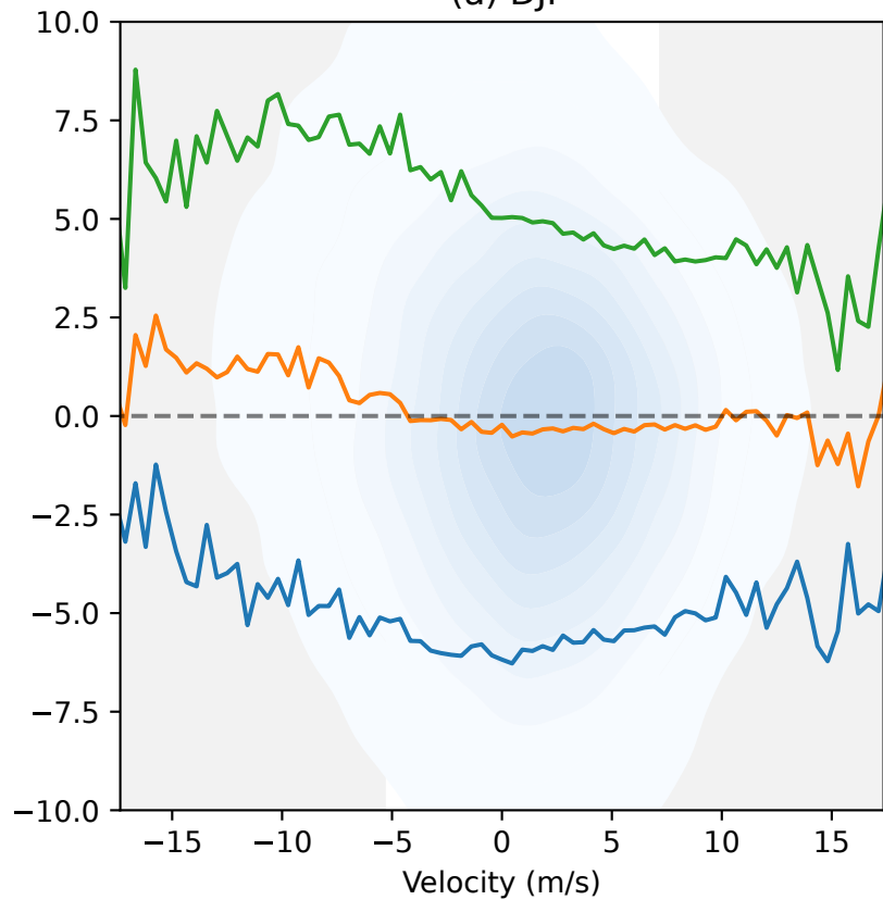
(a) DJF
