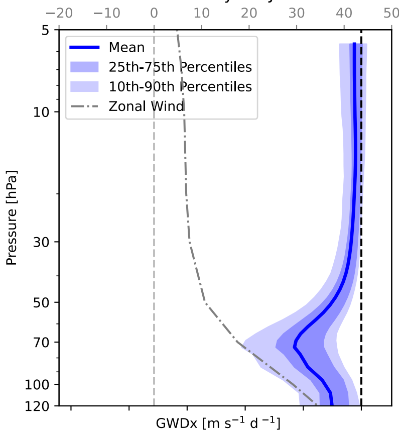
Himalayas DJF
