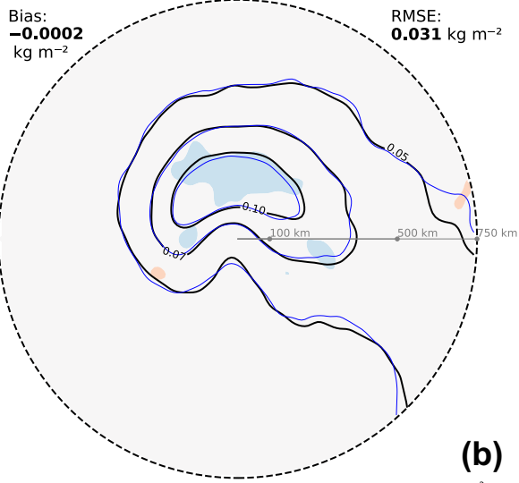
Composite TCIW Bias ( \text{kg m}^{-2} )
