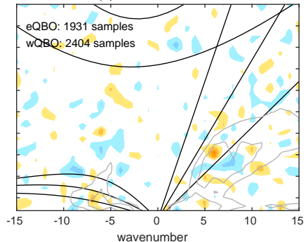
(d) CNRM-CM6-1
