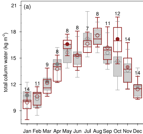
El Nino
