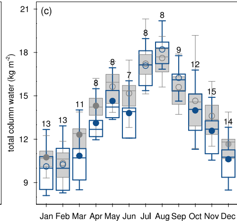
La Nina
