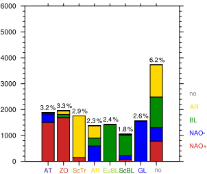
(a) 7+no LC \rightarrow 4 EOF, DJF
