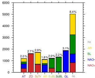
(b) 7+no LC \rightarrow 4 EOF, MAM
