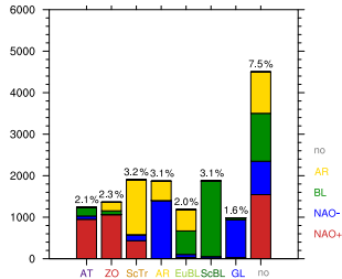
(d) 7+no LC \rightarrow 4 EOF, SON
