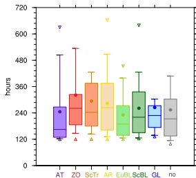
(d) duration (SON)
