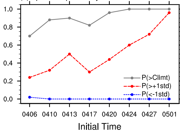
(d) Episode1: probability of Canada Z500 anomaly
