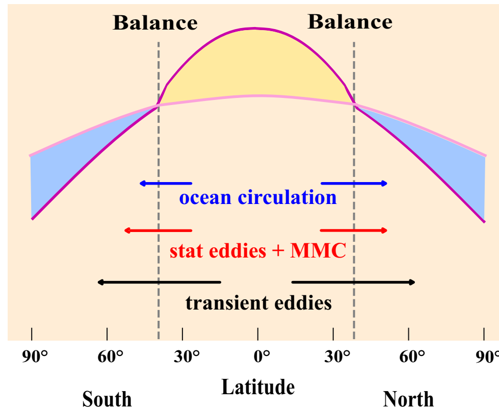
(b) All3
